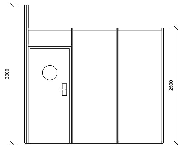
2 RIGHT ELEVATION 1 : 30
